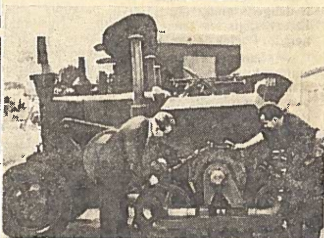
LENKIJOS LIAUDIES RESPUBLIKA. Ščecino žemės ūkio mechanizacijos ir elektrifikacijos institutas išleido pirmuosius pusiauviksčius traktorius. Nauja mašina bus išbandoma laukuose. Nuotraukoje: naujo traktoriaus konstruktoriai inžinieriai Edvardas Jankovskis ir Augustas Kovala. Česliako (Lenkijos Centrinė foto agentūra) nuotr.
